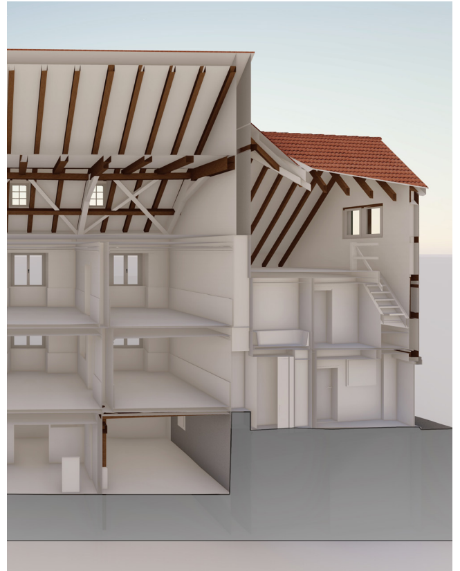
Geschossübergreifende Ansicht aus Längsschnitt
