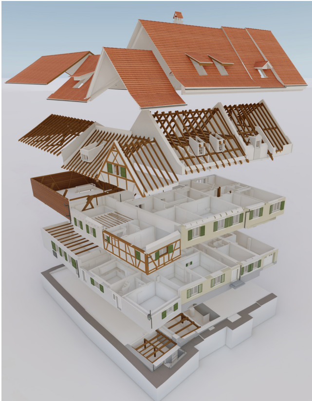
Explosionszeichnung der einzelnen Stockwerke
