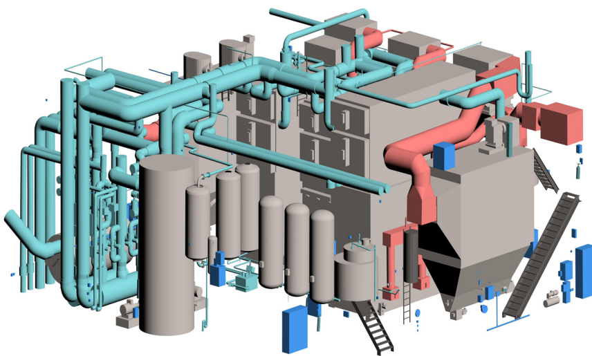
Übersicht 3D-Modell mit der Unterscheidung der einzelnen Objekarten
