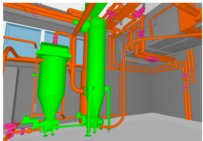
Detail einer 3D-modellierten Anlage
