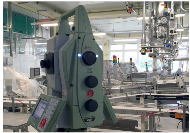
Aufnahme der Produktionsanlage mittels 3D-Laserscanner und Tachymeter
