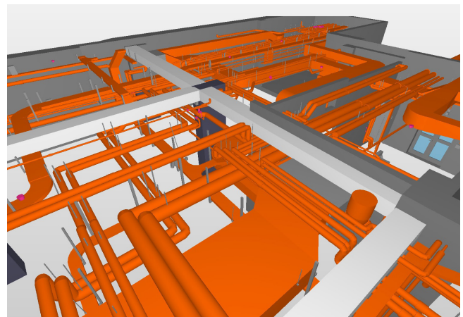
Ausschnitt von einer Decke aus dem 3D-Rohrleitungsmodell
